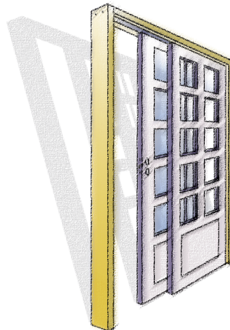
2-FLØYA SKYVEDØRSKARM med eit fast og eit skyvbart felt Type 2 : 70 Tilpassa for 148 mm stender. Dørblad maks. 40 mm tjukt.
