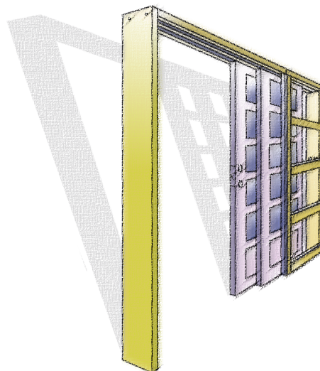
2-FLØYA SKYVEDØRSKARM med eit fast og eit skyvbart felt Type 2 : 70 Tilpassa for 148 mm stender. Dørblad maks. 40 mm tjukt.
